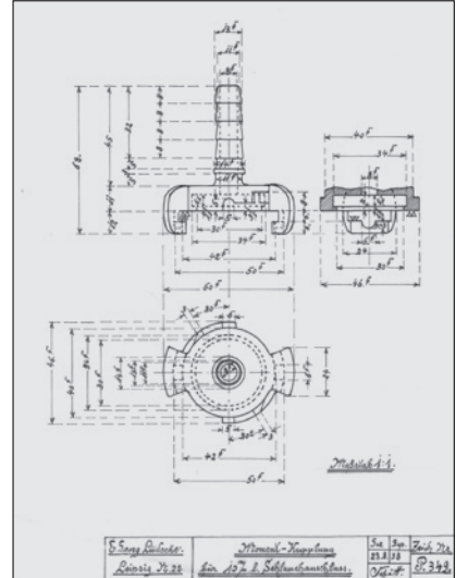
Technische Zeichnung einer Klauenkupplung aus dem Jahr 1938
